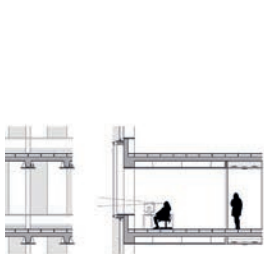
Coupe de principe, éch. 1/50
