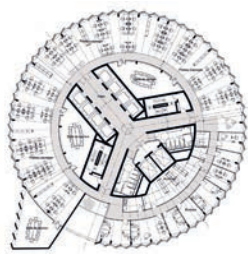
Organisation de la tour de bureaux, éch. 1/200
