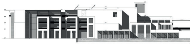
3 CB-Élévation Est Echelle: 1/200e
